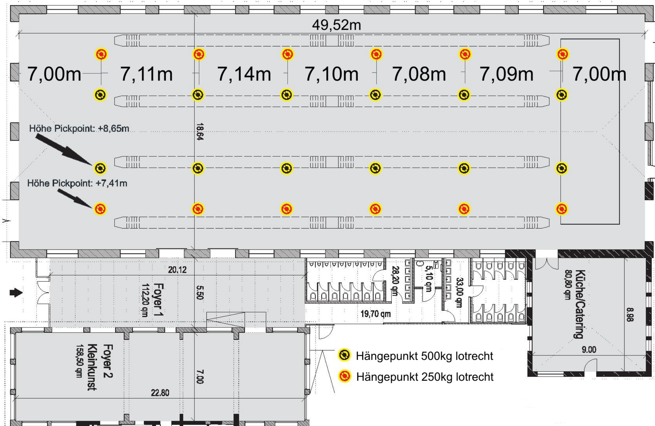
Hängepunkte Phönixhalle
